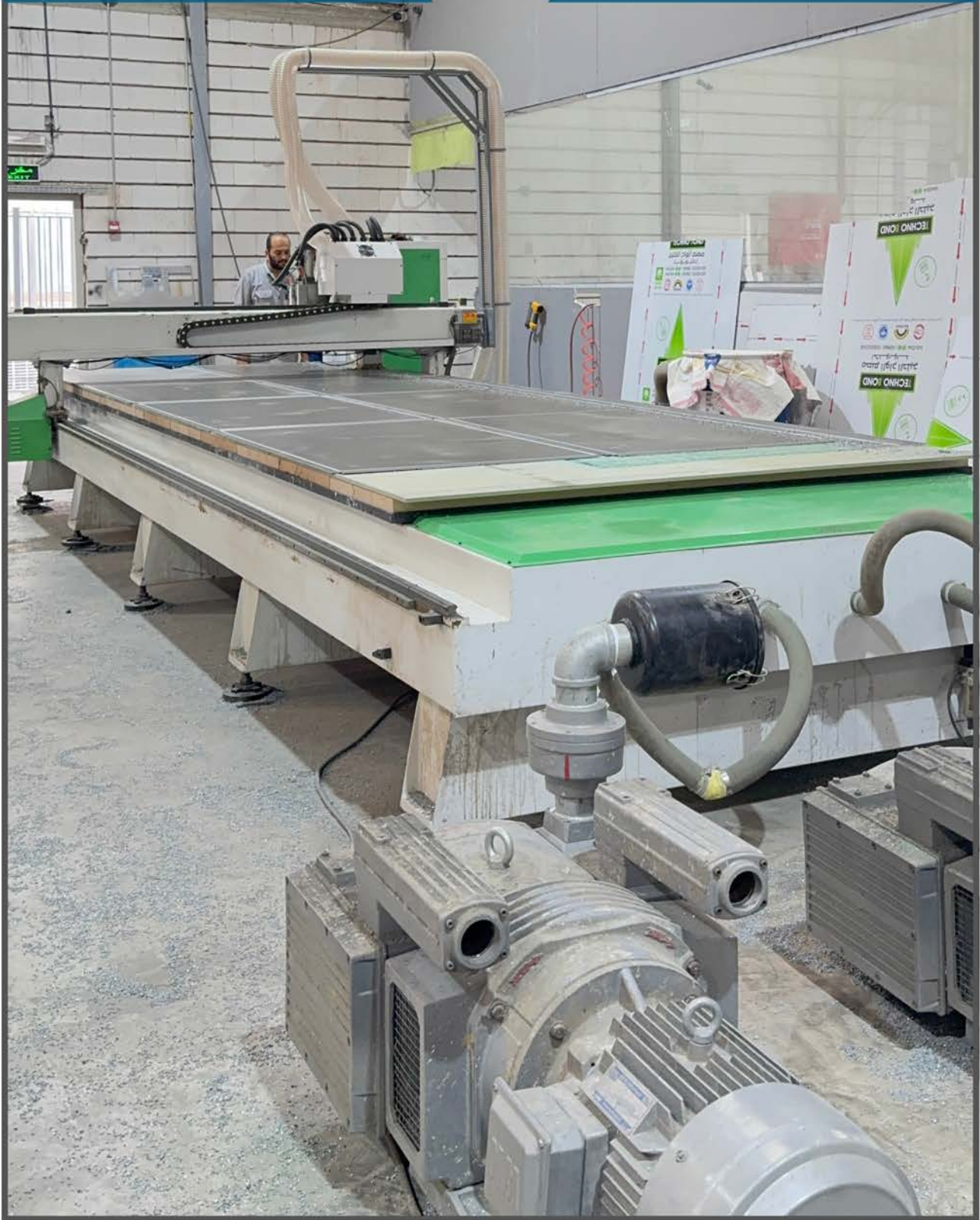
ماكينة CNC Router Heads 3 و 2 x 6
